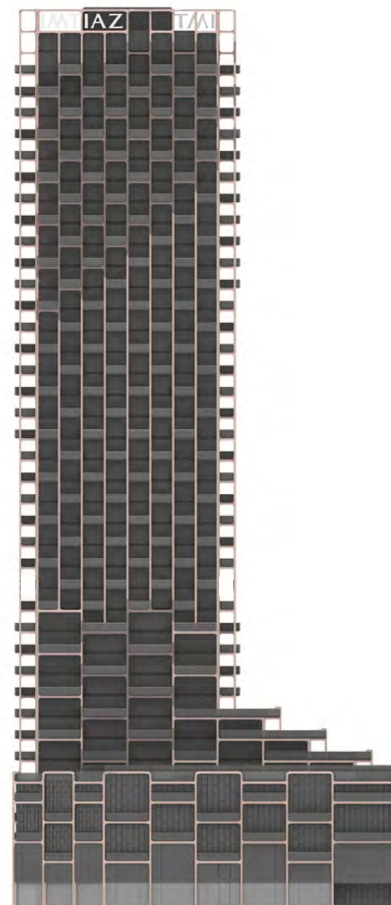
Южный фасад
