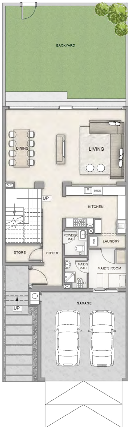
ПЕРВЫЙ ЭТАЖ
